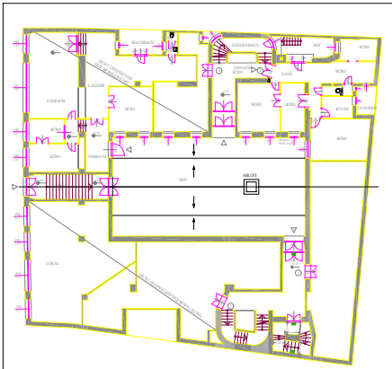
BESTANDSPLAN HOF (OG1) 1988 WIEN, POSTLEINWASSE 11 PROJEKTLEITUNG PROJEKTLEITER PROJEKTLEITERIN PROJEKTLEITERIN PROJEKTLEITUNG PROJEKTLEITER PROJEKTLEITERIN PROJEKTLEITERIN PROJEKTLEITUNG PROJEKTLEITER PROJEKTLEITERIN PROJEKTLEITERIN PROJEKTLEITUNG PROJEKTLEITER PROJEKTLEITERIN PROJEKTLEITERIN PROJEKTLEITUNG PROJEKTLEITER PROJEKTLEITERIN PROJEKTLEITERIN
