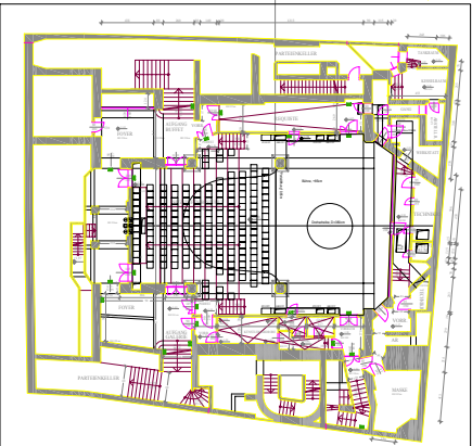
BESTANDSPLAN UG 1988 WIEN, POSTLEINWASSE 11 PROJEKTLEITUNG PROJEKTLEITER PROJEKTLEITERIN PROJEKTLEITERIN PROJEKTLEITUNG PROJEKTLEITER PROJEKTLEITERIN PROJEKTLEITERIN PROJEKTLEITUNG PROJEKTLEITER PROJEKTLEITERIN PROJEKTLEITERIN PROJEKTLEITUNG PROJEKTLEITER PROJEKTLEITERIN PROJEKTLEITERIN PROJEKTLEITUNG PROJEKTLEITER PROJEKTLEITERIN PROJEKTLEITERIN
